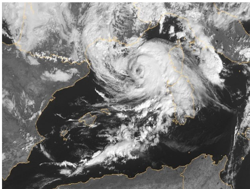
Medicà del 8 de novembre de 2011 font: EUMETSAT)
