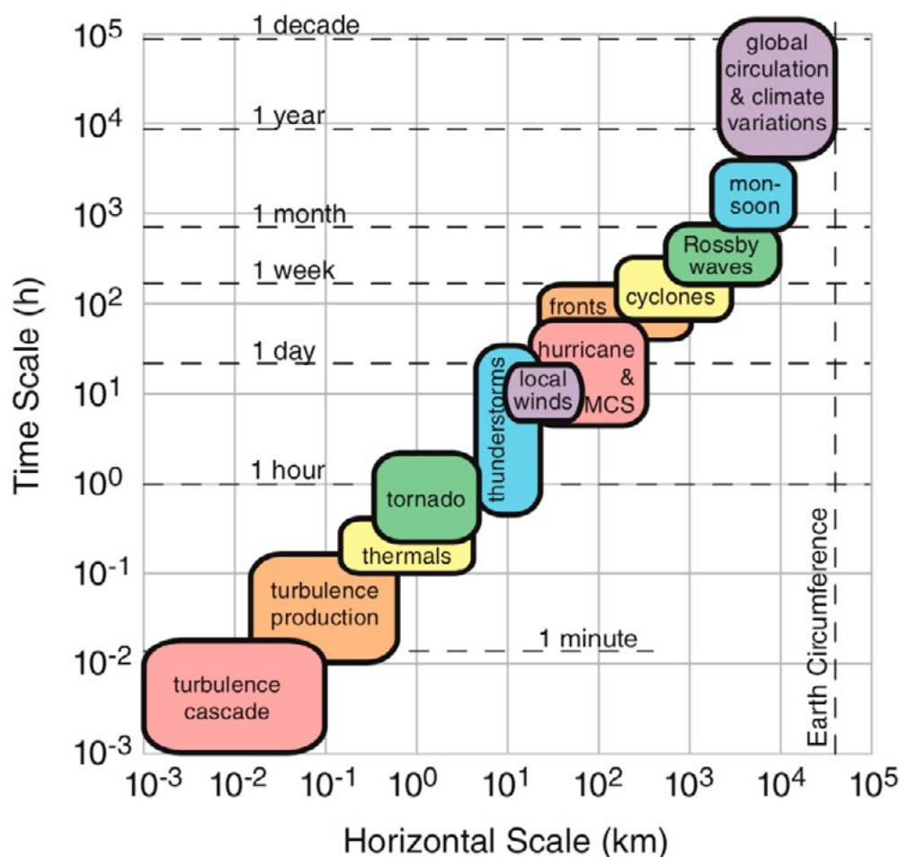
Diagrama d'escales horitzontals i temporals de les circulacions atmosfèriques (font: Stull 2017)
