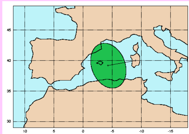
Sardinia
